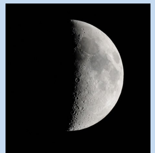
月齢7の月
