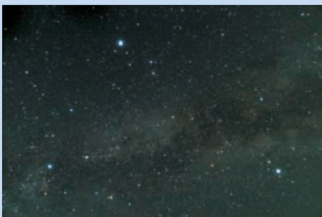
夏の天の川と天の川 （中央上：ベガ、右下：アルタイル、左下：デネブ）
